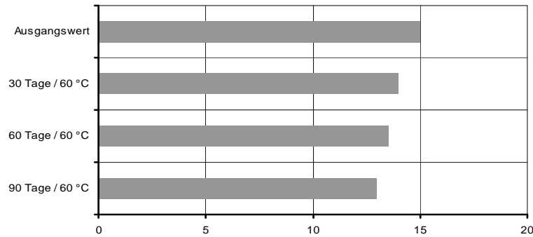
Durchschnittliche Scherfestigkeit bei Überlagerung (N/mm 2 ) bezogen auf Wärmealterung
