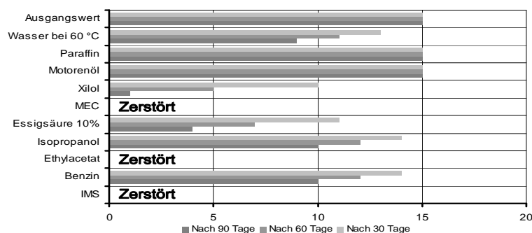
Durchschnittliche Scherfestigkeit bei Überlagerung (N/mm 2 ) bezogen auf die Alterung der Wirkstoffe
